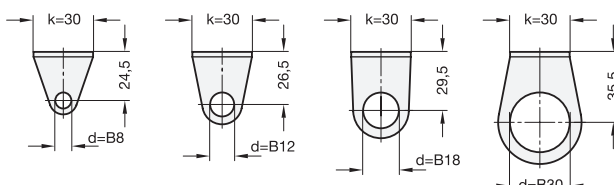
Draufsichten für verschiedene Bohrungs- \varnothing d
