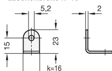
Draufsichten für verschiedene Bohrungs- \varnothing d
