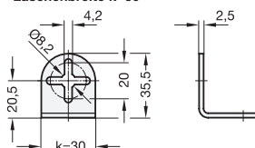
Draufsichten für verschiedene Bohrungs- \varnothing d
